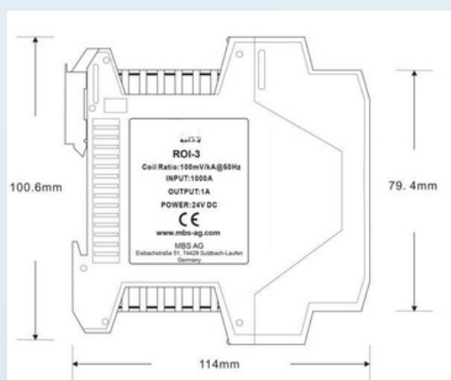
Abbildung 9: Abmessungen des ROI-3
