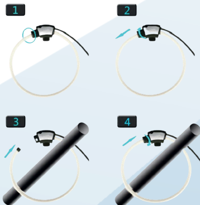
Abbildung 6: Montage der FASK
