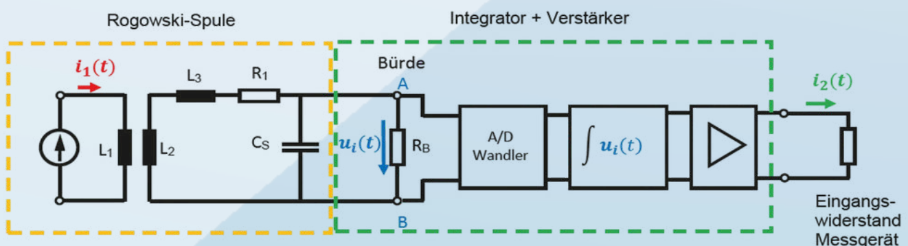
Abbildung 3: Elektrisches Ersatzschaltbild Rogowski-Spule + 1 A Integrator
