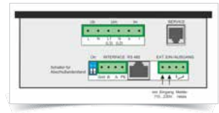
Abb.: Prophi® 7 Schnittstelle
