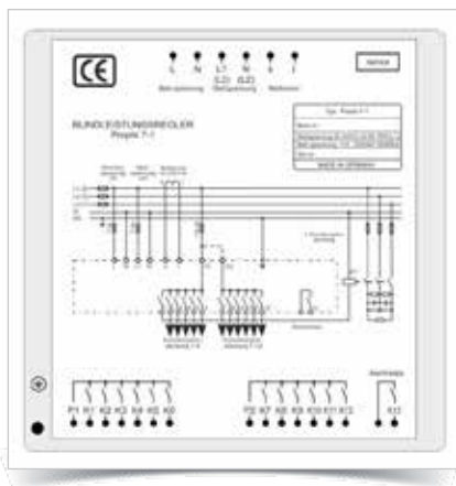
Abb.: Prophi® 7 Rückseite
