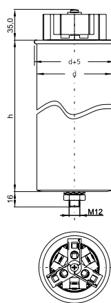
Kondensator mit Anschlussstück ASS 2 d = 85 mm
