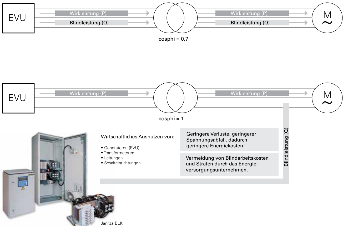
Abb.: Wirk- und Blindleistung im Leitungsnetz mit Kompensation
