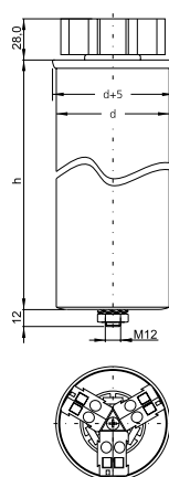
Kondensator mit Anschlusstück ASS 1 d = 60 / 70 mm
