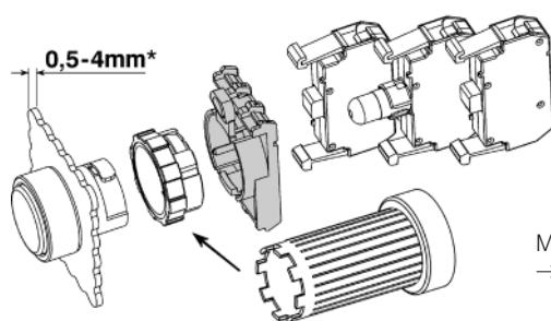
Kuppelstück B3M
